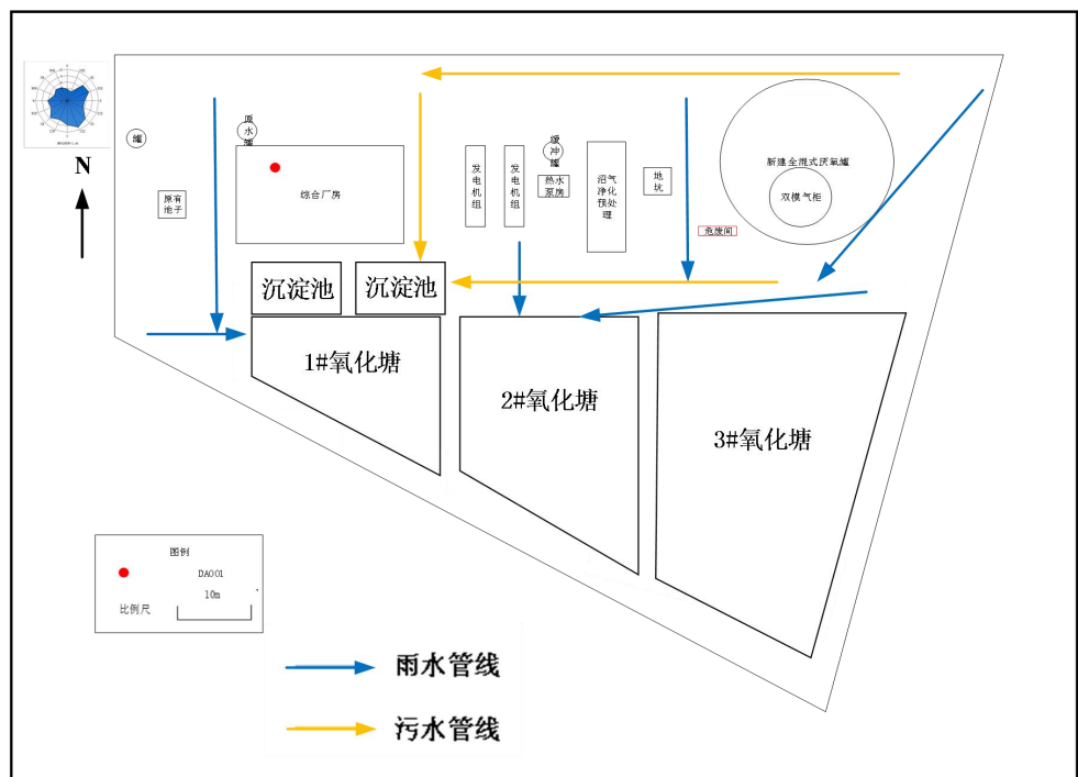
图 4-4 项目雨污管线及排放去向分布图
