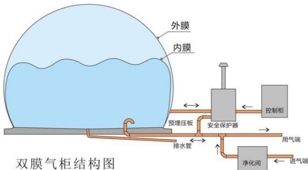
图 3-7 双膜气柜原理图
