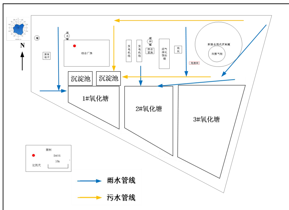
图 3-3 项目平面布置图
