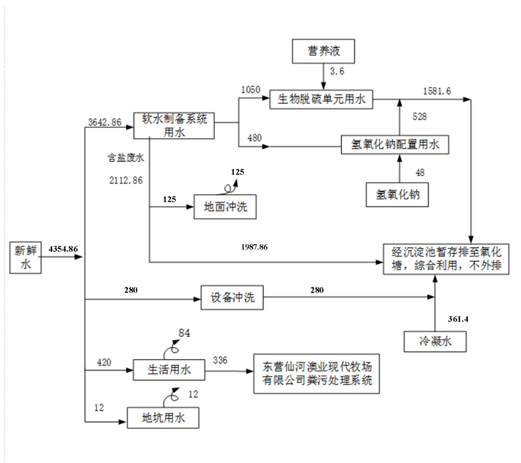
图 3-4 项目实际水平衡情况图
