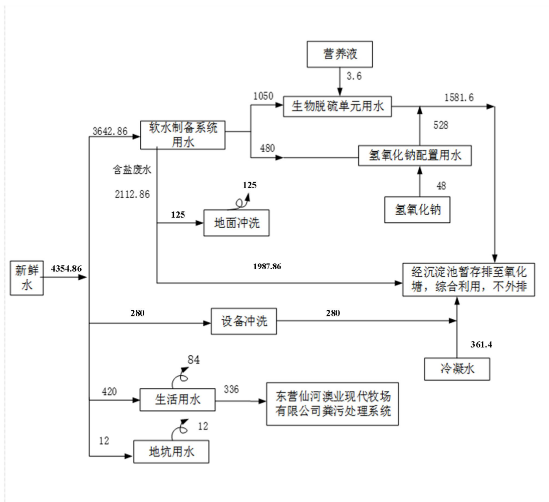
图 4-2 项目水平衡图 (t/a)
