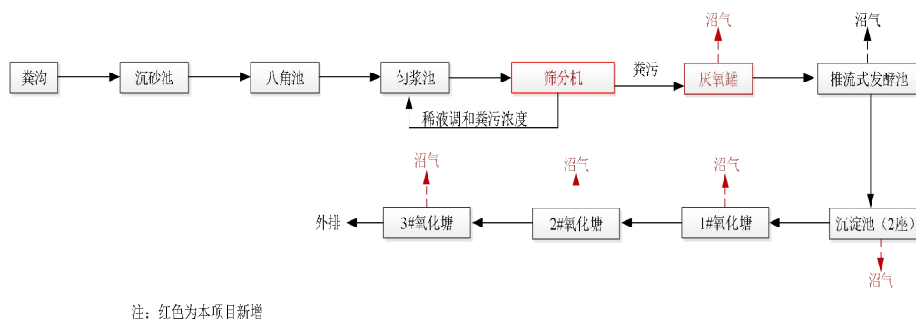
图 3-5 粪污处理工艺流程图
