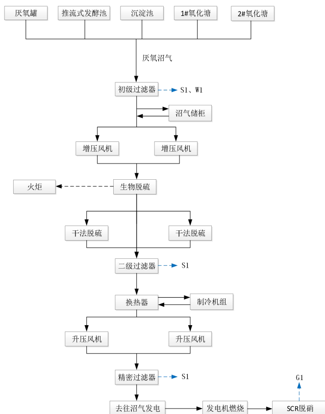
图 3-6 沼气发电生产工艺流程图
