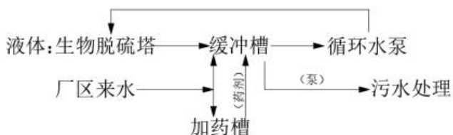
图 3-8 脱硫工艺示意图
